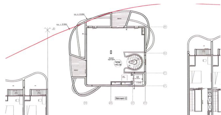
ELLA ETAGE 6 | Bâtiment C-Etage 3 -éch: 1/100e
