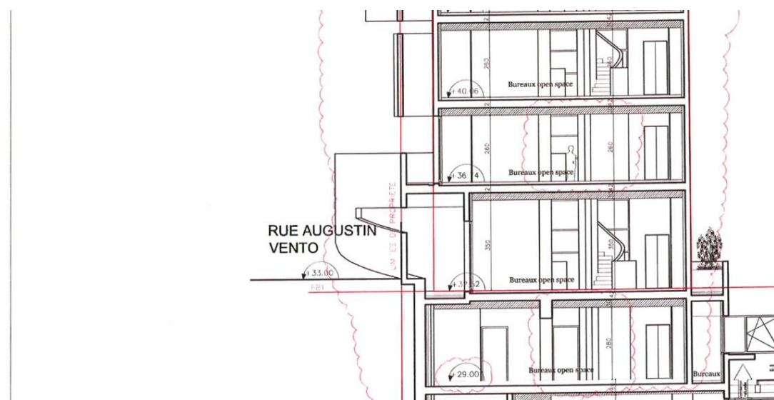
ELLA ETAGE 6 | Bâtiment C-Etage 3 -éch: 1/100e
