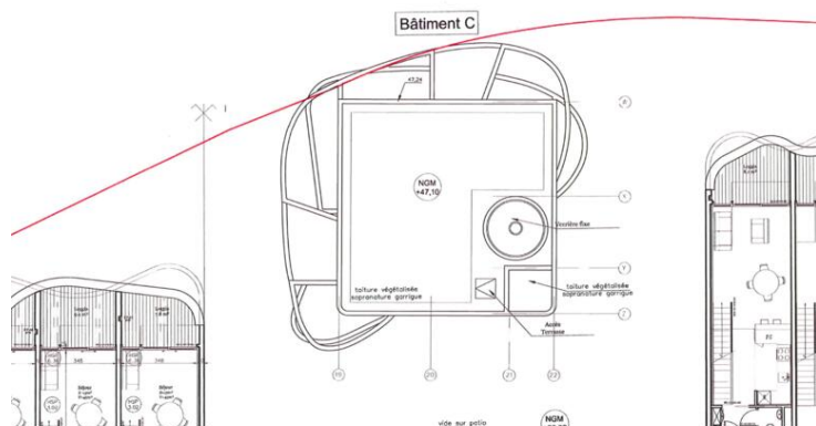
ELLA ETAGE 7 | Bâtiment C-Toiture-éch: 1/100e
